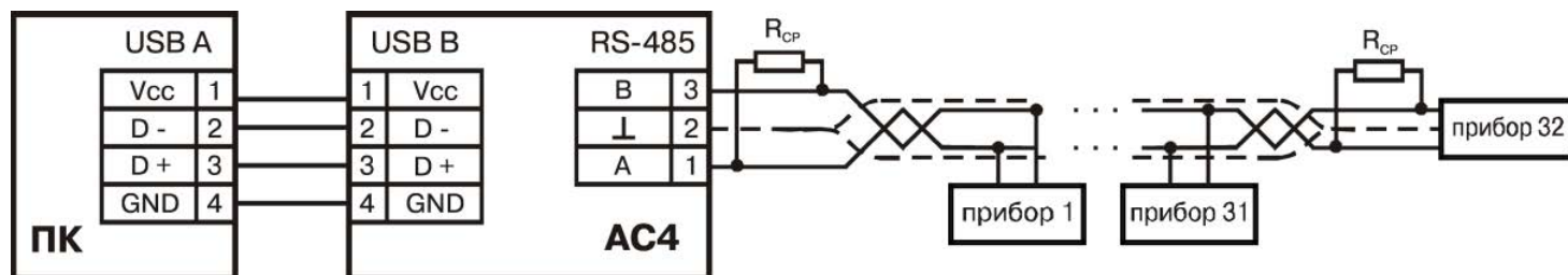
Рисунок 3 - Схема подключения прибора
